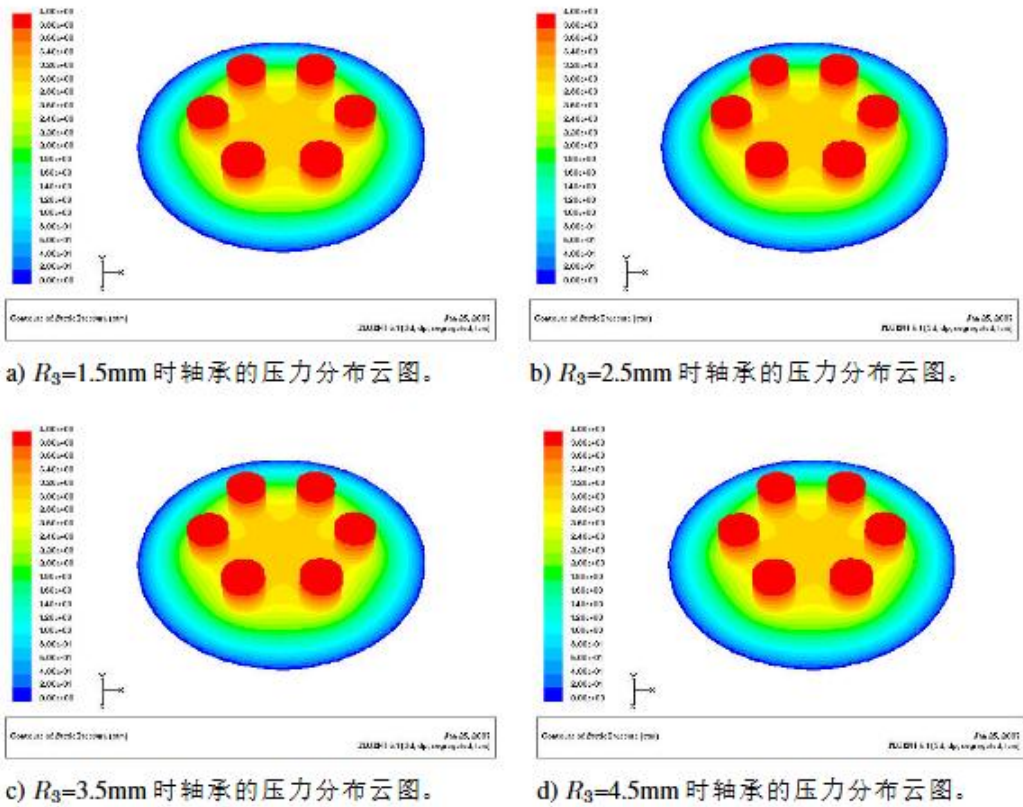
图 4-2 局部多孔质圆柱塞半径不同时轴承的压力分布云图。
